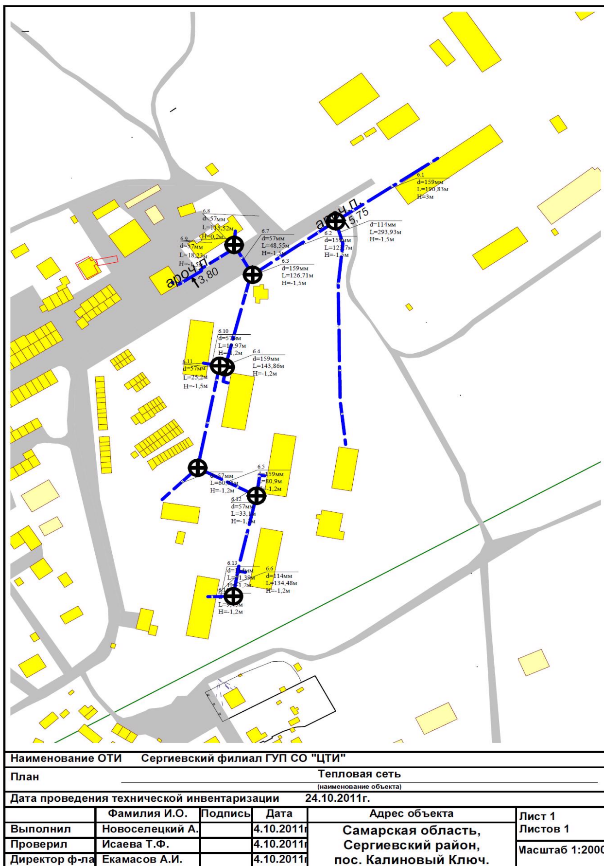
Рис. № 6 - Схема тепловых сетей от Центральной котельной п. Калиновый Ключ
